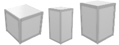
A B C Width Height Depth A) 500mm x 500mm x 500mm B) 500mm x 500mm x 750mm C) 500mm x 500mm x 1000mm
